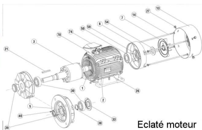
Eclaté moteur
